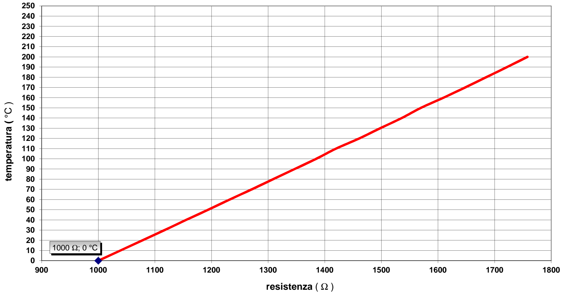
COD 1.033678 grafico resistenza-temperatura sonda Pt 1000 collettore - bollitore Brahma
