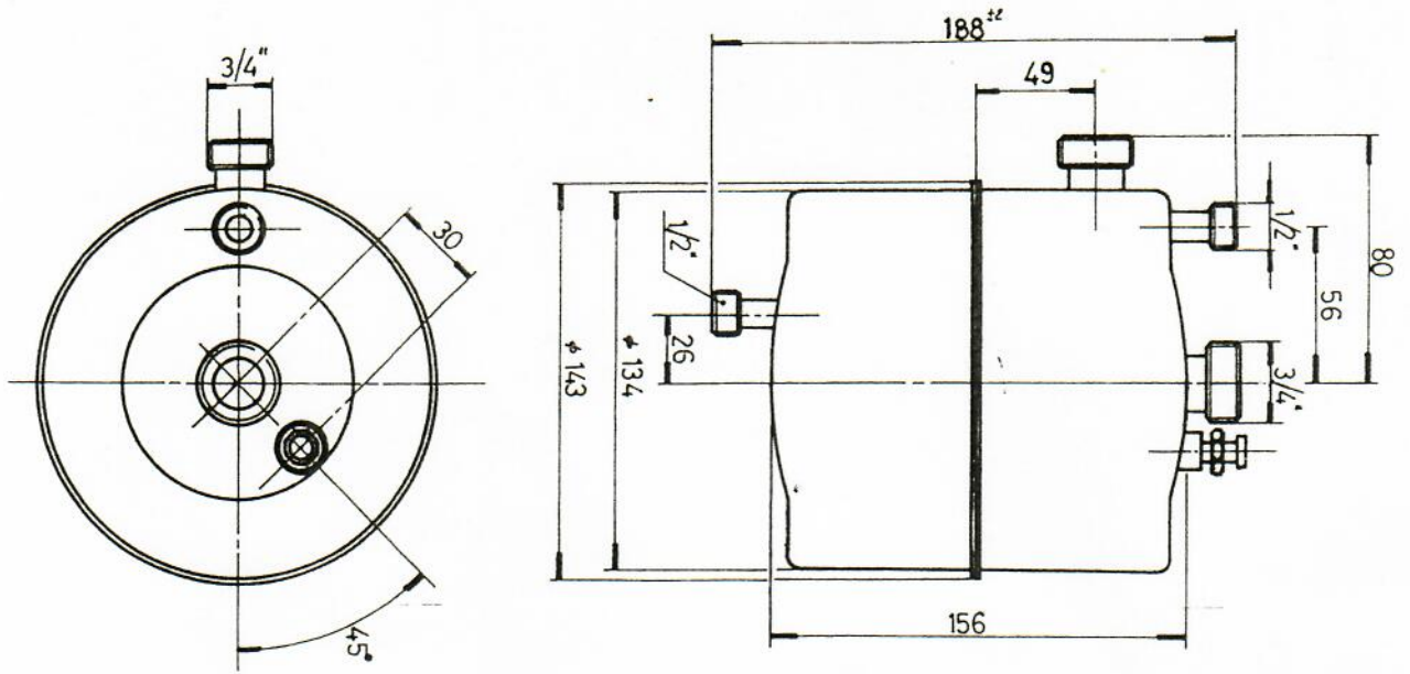
MOD. 5/8 PER CALDAIA BALTUR
