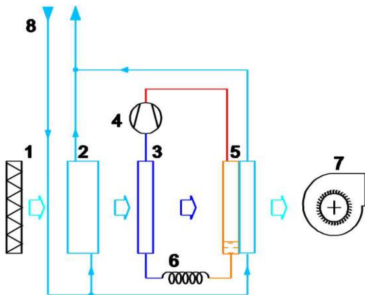
Fig. 1 Schema del deumidificatore
